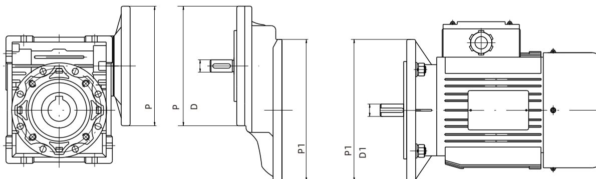
PC+WMRV 组合型减速机组合方式 Combination of PC+WMRV reducer
