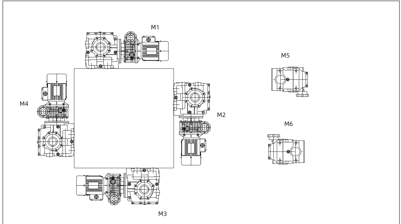
MB无级与WS系列组合安装方式
