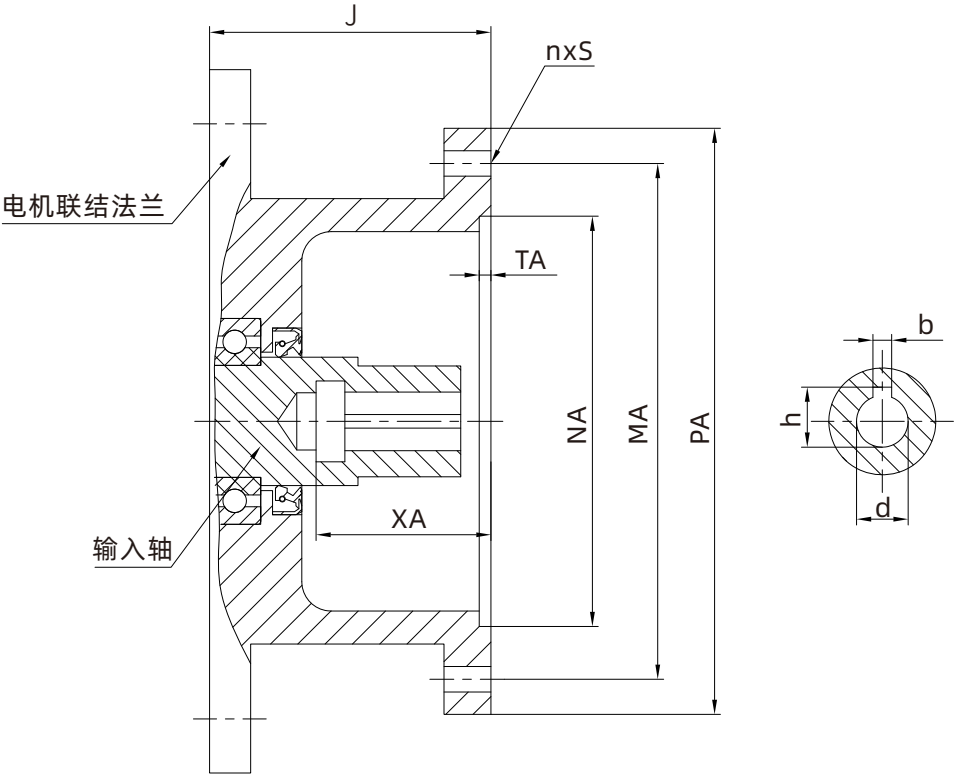
十九、配Y系列电机时联接法兰尺寸图表
