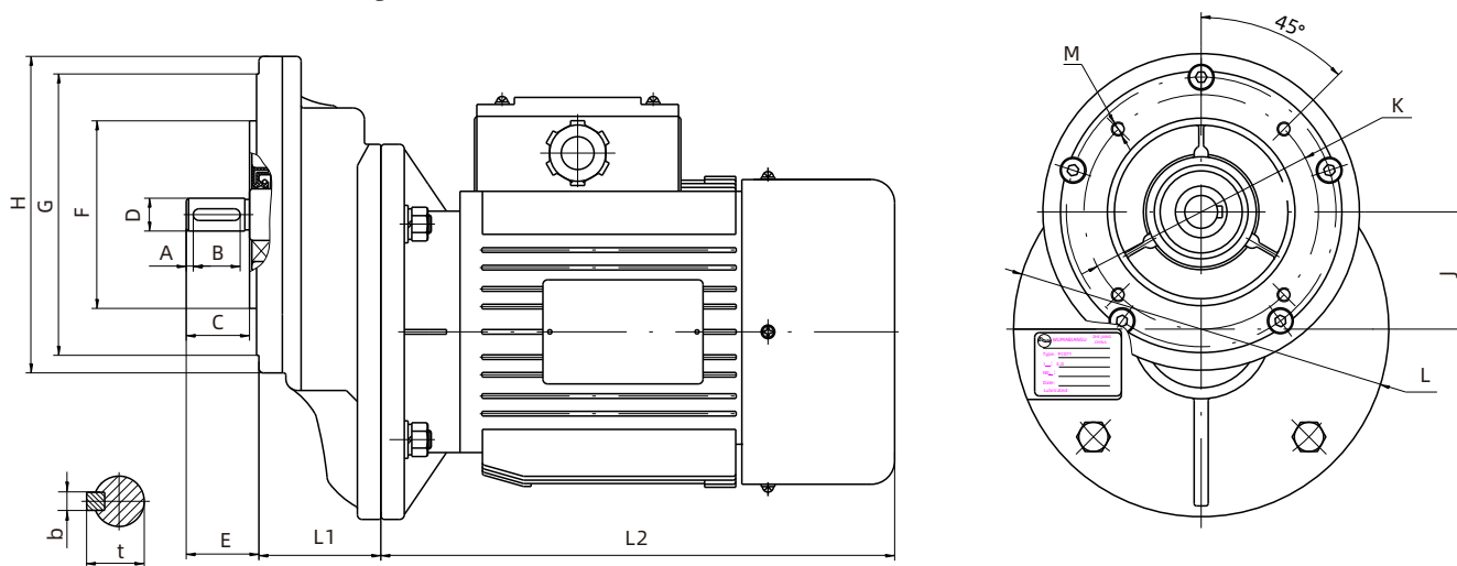
PC系列减速机外形尺寸图
